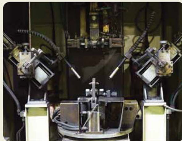
용접 전용기 / Exclusive welding machine / 溶接専用機
